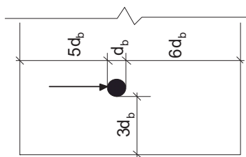
Σχ. Σ6.6: Ορισμός επικάλυψων βλήτρου
